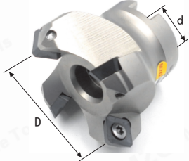
KM Çelik 45° Yüz Freze Kesici KM Steel 45° Face Milling Cutter
