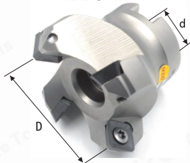
KM Staal 45° Face Fräsing KM Steel 45° Face Milling Cutter
