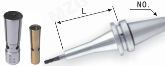
SDC Geri Çekilmiş Collet Toolholder SDC Back-Pull Collet Toolholder
